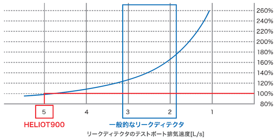
排気速度と応答速度(5L/sを100%とした比)
