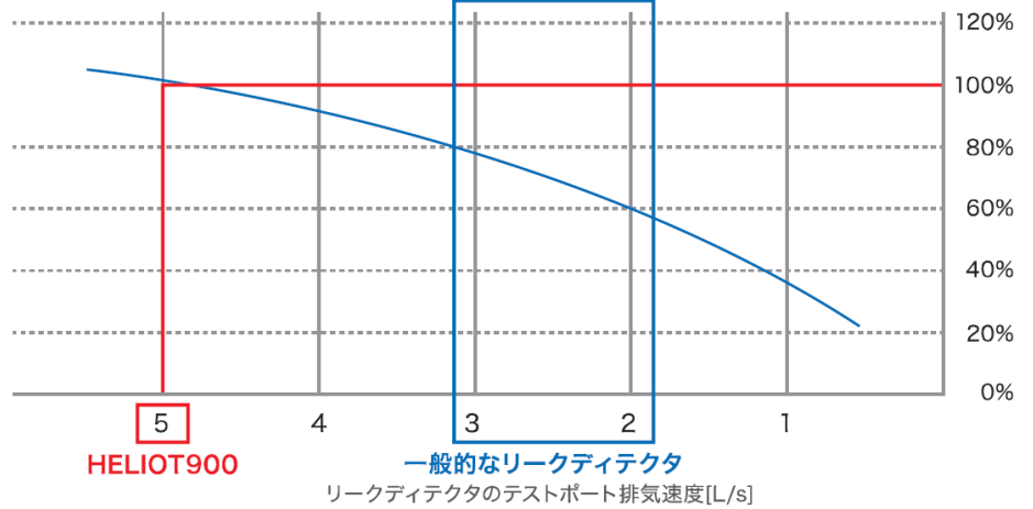
排気速度と測定値(5L/sを100%とした比)
